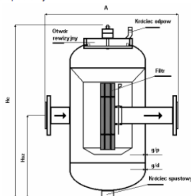
Typ – IOW kolnierzowy
